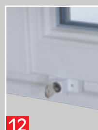
Verrouilleur à clé pour condamnation de l'ouverture à la française Coloris blanc gris et aspect inox. Disponible uniquement avec ferrage oscillo-battant
